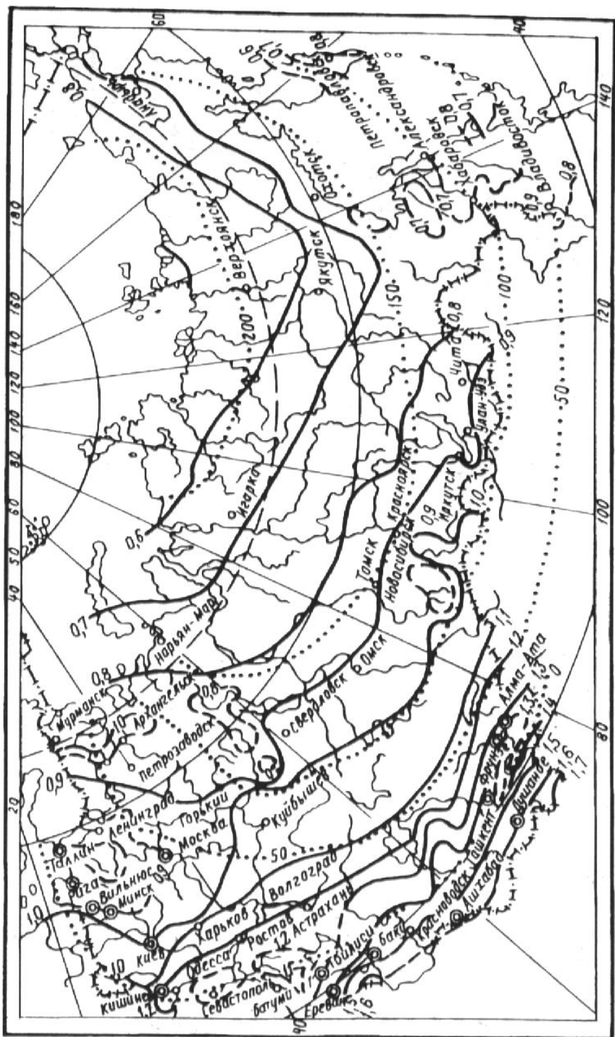
Черт.3. Климатические коэффициенты для определения величины нагрузки на иловые площадки (сплошные и пунктирные линии) и продолжительности периода намораживания на иловых площадках, дни (точечные линии)
