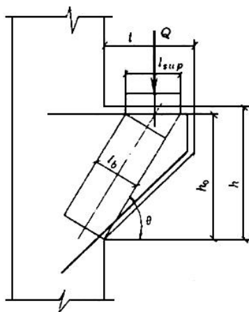
Черт.11. Схема для расчета коротких консолей
