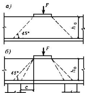
Черт.16. Схемы для расчета железобетонных элементов на продавливание
