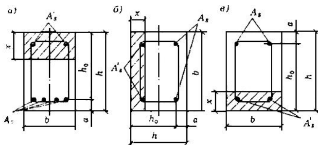
Черт.14. Схема расположения сжатой зоны пространственного сечения
