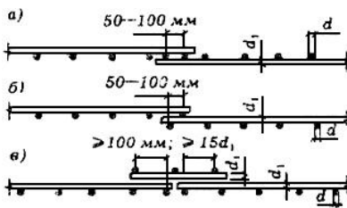
Черт.26. Стыки сварных сеток в направлении распределительной арматуры
