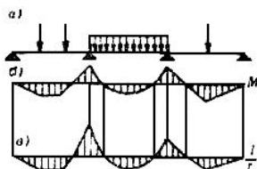
Черт.21. Эюры изгибающих моментов и кривизны для железобетонных элементов постоянного сечения
